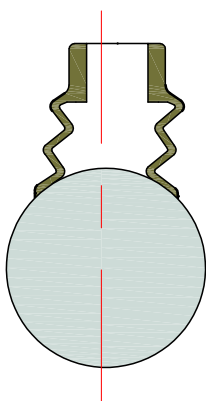
▶ 原2段波纹管吸取形状
