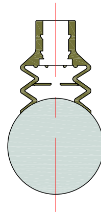
▶ 横向负荷2段波纹管吸取形状
